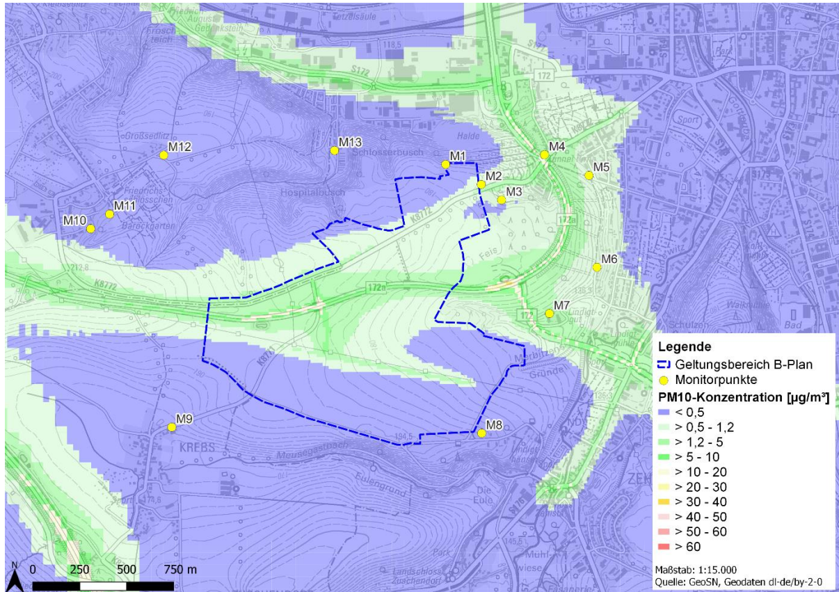
Abbildung 11: verkehrsbedingte Immissionszusatzbelastung (IZ) der PM 10 -Konzentration im Prognose-Planfall mit Berücksichtigung von Kaltlufteinflüssen
