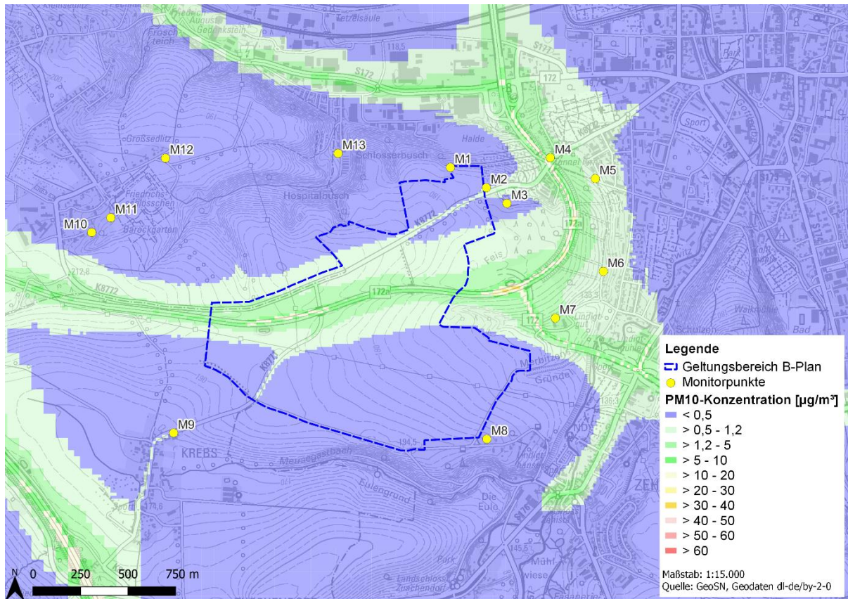
Abbildung 10: verkehrsbedingte Immissionszusatzbelastung (IZ) der PM 10 -Konzentration im Prognose-Nullfall mit Berücksichtigung von Kaltlufteinflüssen
